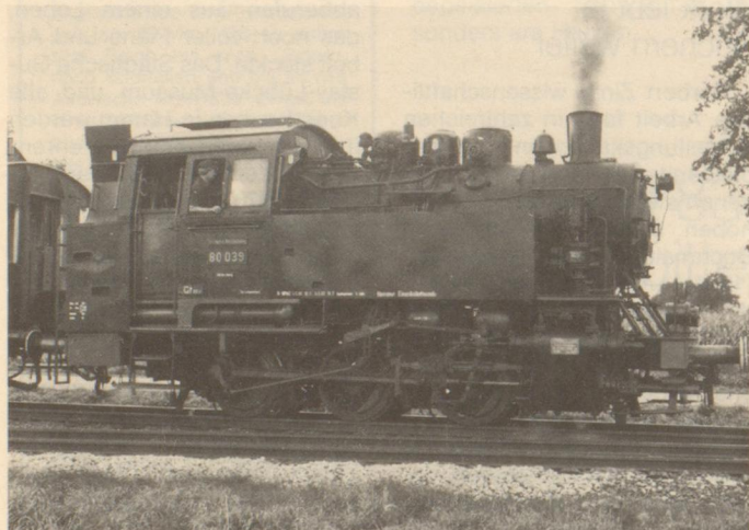
Sie hält die Museumsbahn unter Dampf: Die Lokomotive 80039 der Hammer Eisenbahnfreunde
