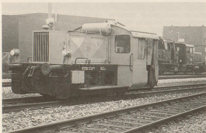
Die „Köf II“ ist jetzt im Eigentum der Hammer Eisenbahnfreunde.
