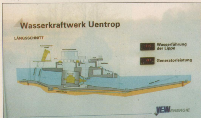
Längsschnitt des Wasserkraftwerkes
