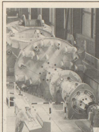
Die größte Verseilmaschine der Welt wird am 9. Februar von der Thyssen-Draht AG Hamm in ihrem Werk in Gelsenkirchen in Betrieb genommen. Auf dieser Maschine können Drahtseile bis zu 305 Millimeter Durchmesser und in Stückgewichten bis zu 200 Tonnen gefertigt werden.
