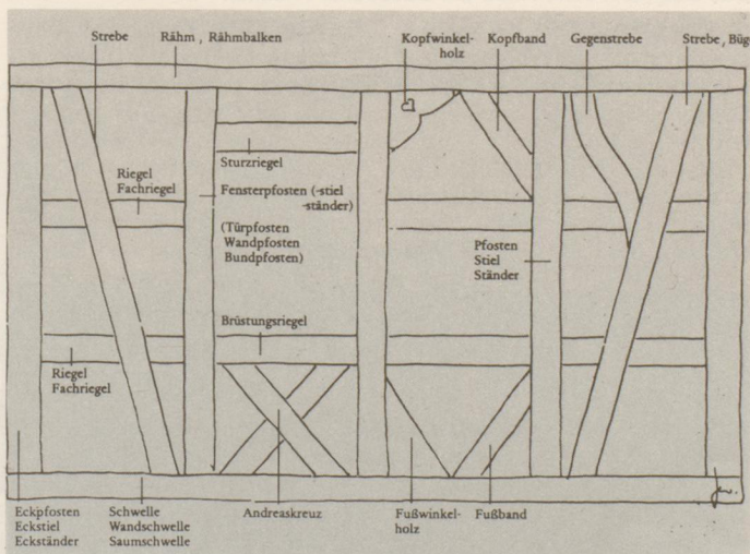
Fachwerkhölzer und ihre Bezeichnungen innerhalb der Baukonstruktion.
