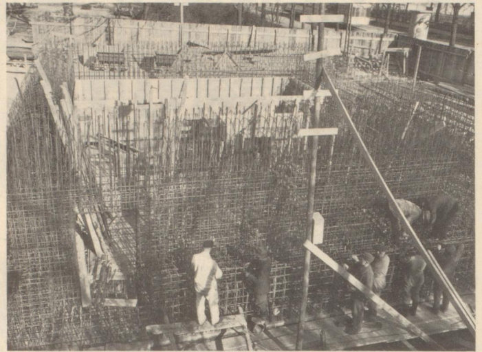
Bunkerbau an der Ostenallee am Eingang des Kurparks im März 1941.
