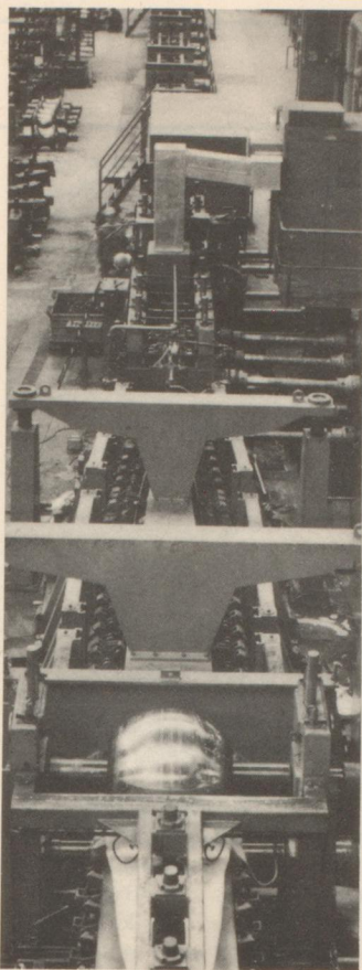
Aggregat für das Einformen vom Band zum Schlitzrohr.
