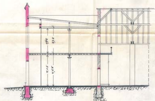
Schnitt-B
