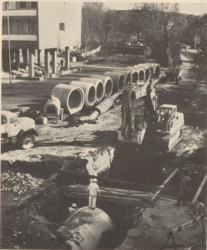
Als große Tiefbaustelle bietet sich der Südring zwischen Westentor und Goethestraße. Nach der Verlegung der riesigen Betonrohre für den neuen Hauptsammler (unser Bild) erfolgt der Ausbau der Fahrbahn.
