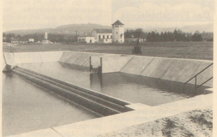
Filterbecken mit Kaskade zur Sauerstoffanreicherung.
