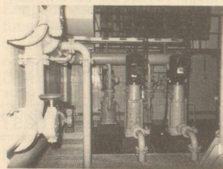
Innenansicht der Wasserdruckerhöhungsanlage Heessen.
