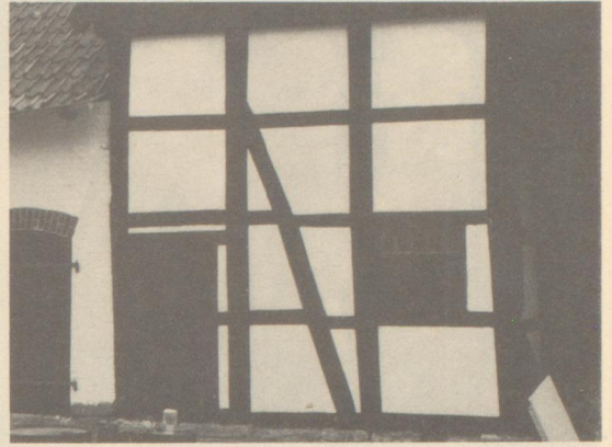
Die Restaurierung des Loh-Hofs: Das Lehmstampfgefach war Ende des 19. Jahrhunderts durch Weichbrandziegel ersetzt, das Balkenwerk mit brauner Ölfarbe überstrichen und die Stalltür zugemauert worden. Das rechte Bild zeigt die fertige Vorderfront mit verputzten und gestrichenen Feldern. Die Balken wurden mit einem hochwertigen Holzschutzmittel behandelt, Tür und Fenster erneuert.
