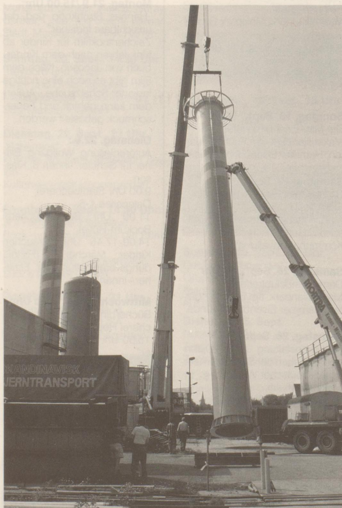
Schwere Hebekräne nehmen die 32 Meter langen Kamine an den Haken.
