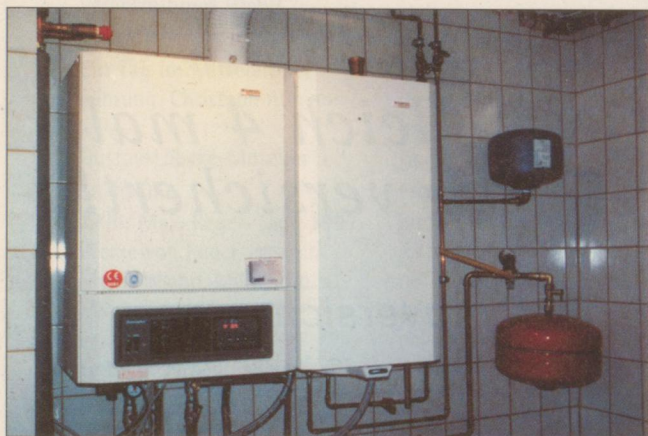
Eine moderne Erdgas-Brennwertanlage mit Brauchwasserspeicher
