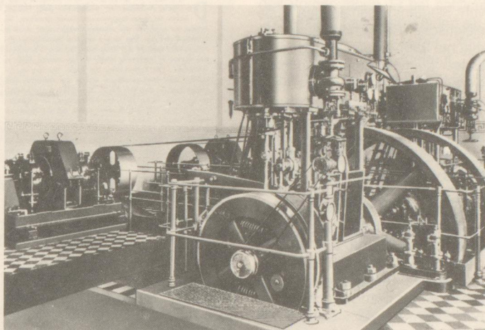
Fig. 8. Maschinennast der Zentrale Hamm i. W.
