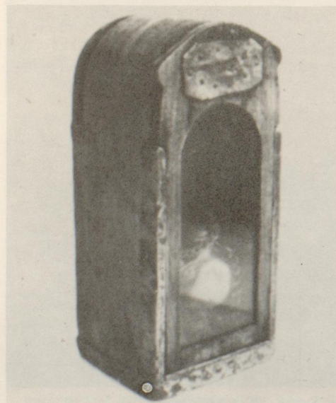
Freiberger Blende aus dem sächsischen Erzgebirge.
