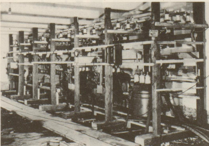
Dieser Hochspannungsschaltanlage wäre ein Platz im Museum sicher.
