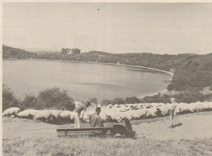
Kratersee in der Vulkaneifel.
