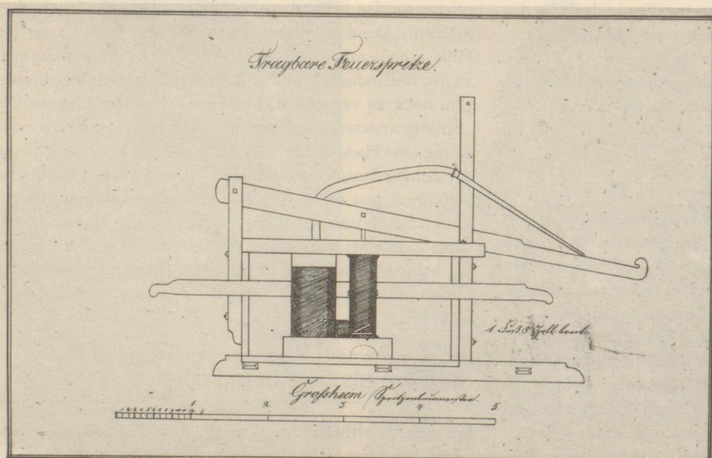
Modell einer tragbaren Feuerspritze von 1799.
