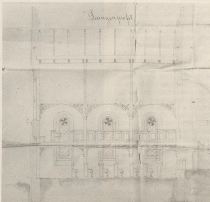
Hammer Synagoge, Längenprofil.
