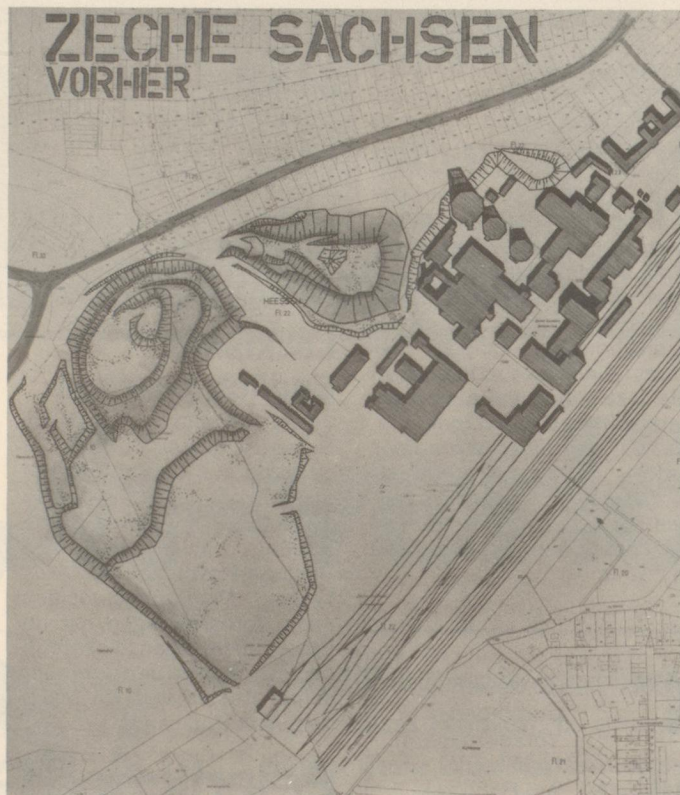
1976 wurde die Zeche Sachsen in Hamm-Heessen stillgelegt. Der Plan zeigt den Bestand an Halden (links) und Gebäuden (rechts) zum Zeitpunkt der Stilllegung.
